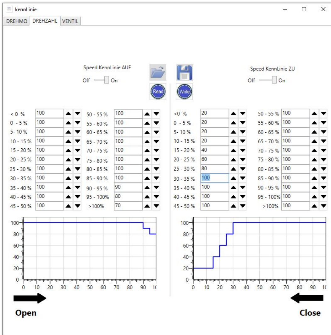
Bild 63: Drehzahl Kennlinie
