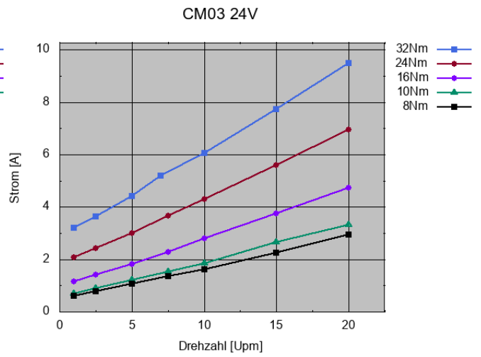
Bild 93: Stromaufnahme der 24 VDC-Version
