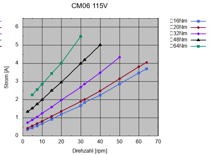
Bild 96: Stromaufnahme der Standard-Version
